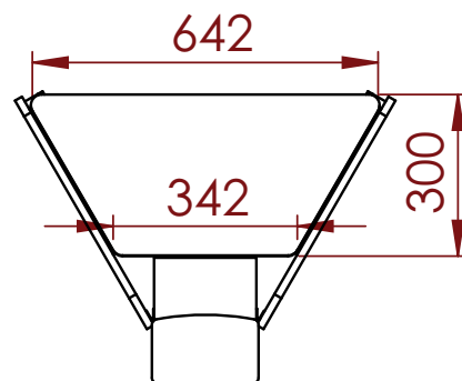
Dimensions de la tablette
